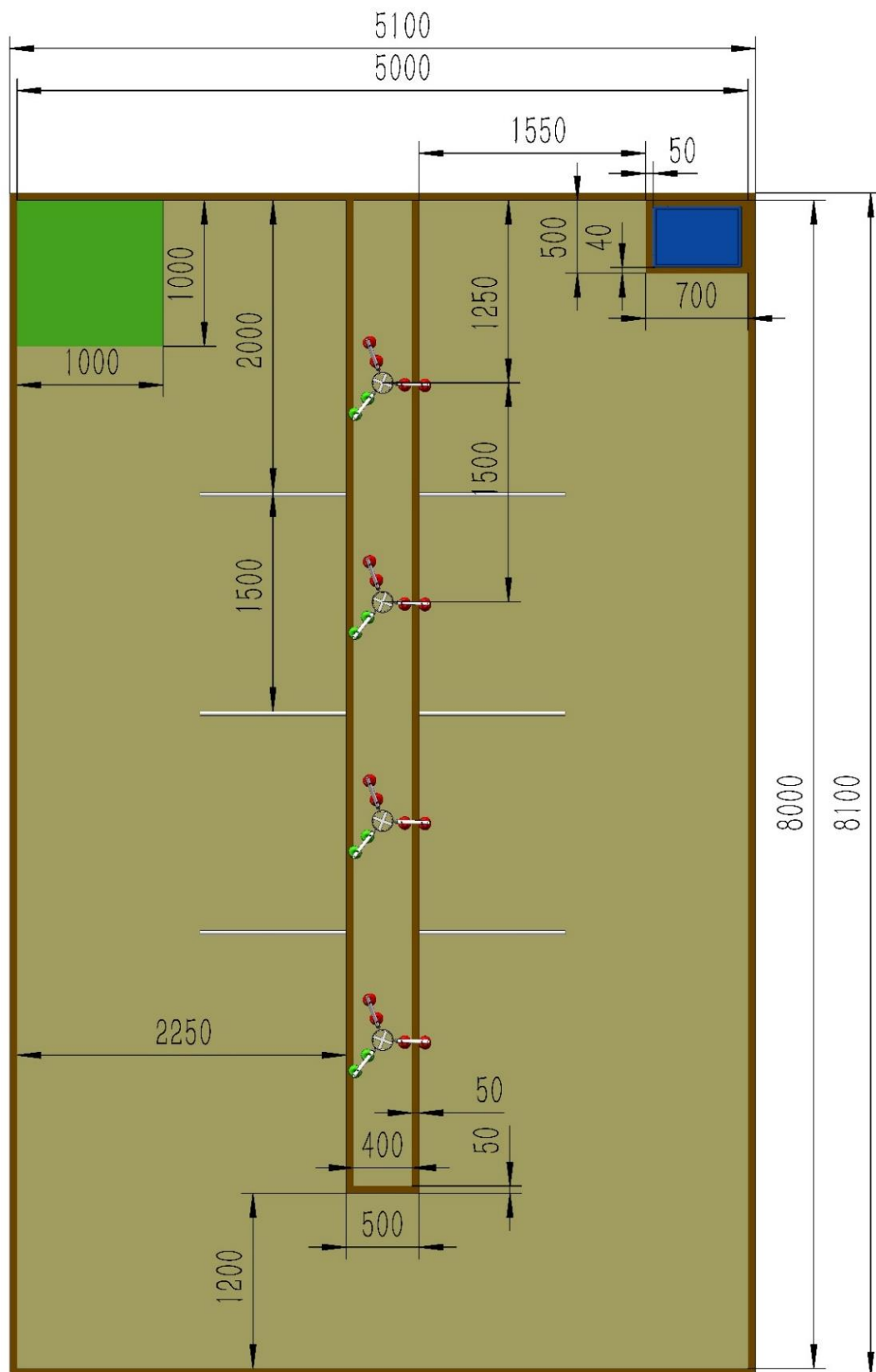
图 2 场地俯视图
