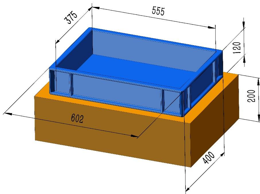
图 4 果实放置区
