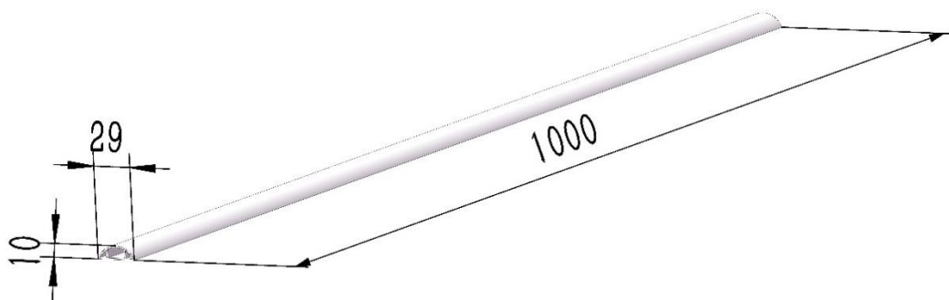
图 3 减速带
