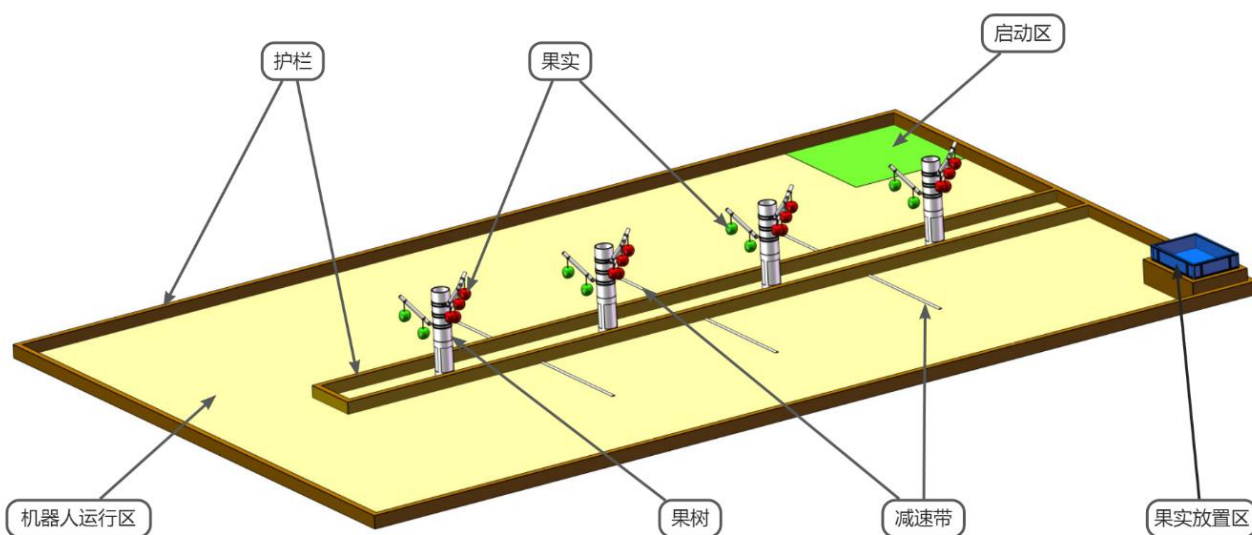
图 1 场地三维图
