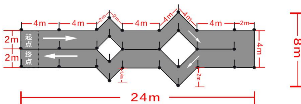
室外搭建 64m (例 1)
