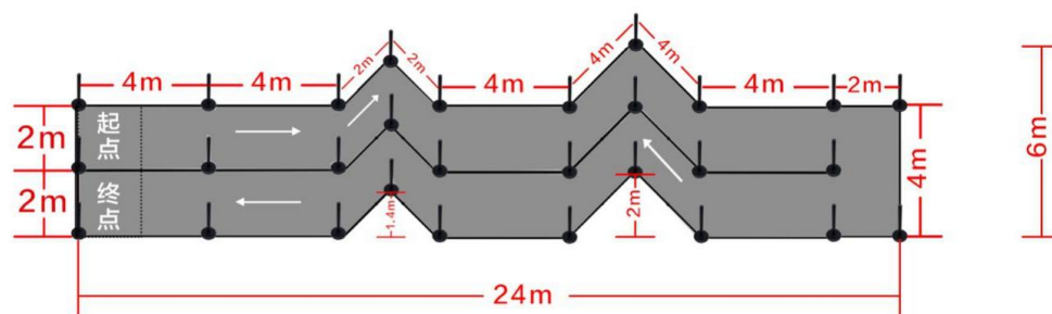
室内搭建 64m (例 2)
